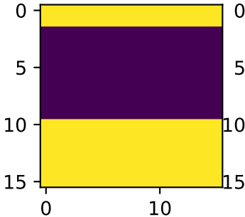
T = 0.5
